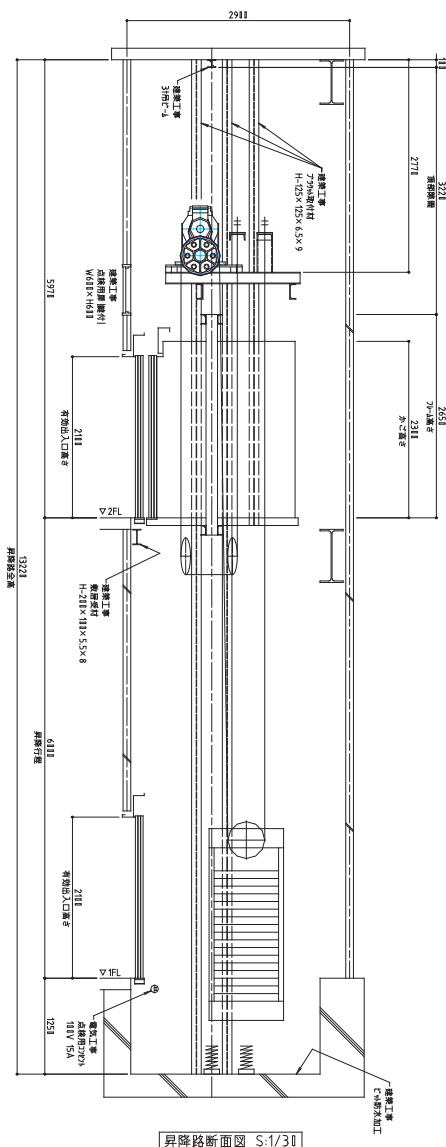
昇降路断面図 S:1/31
