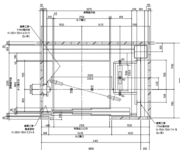
昇降路平面図 S:1/25
