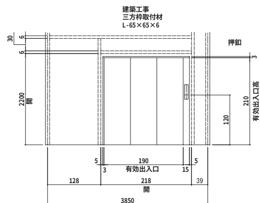
出入口正面図
