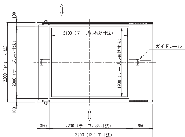
A-A矢視図
